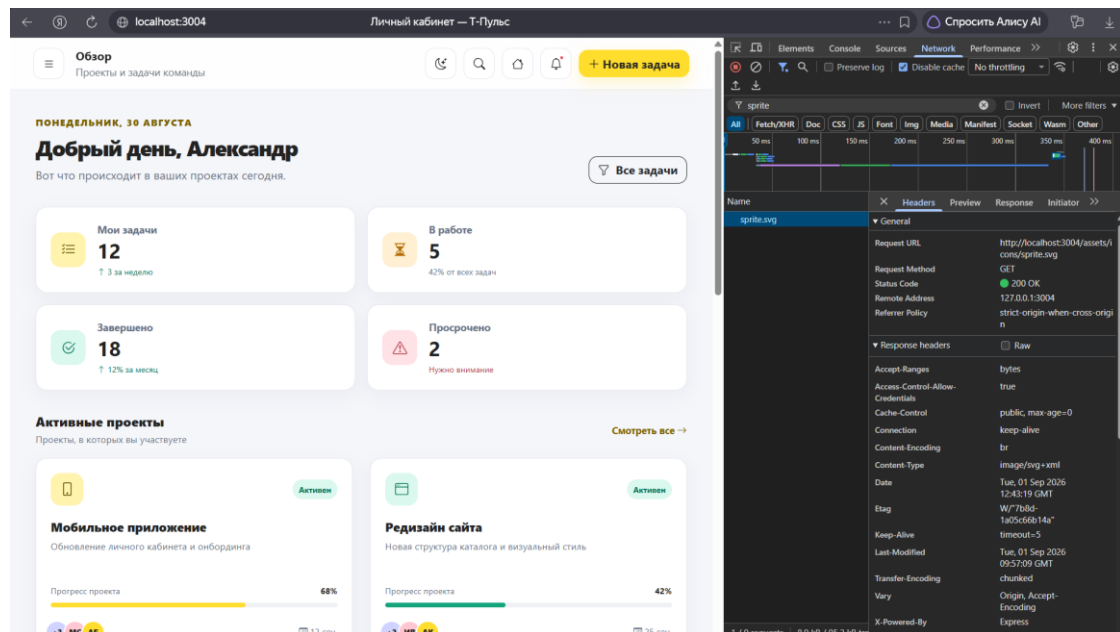
Рисунок 6 - Успешная загрузка sprite.svg в панели Network
